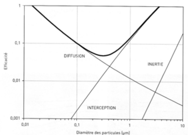
Figure 15 : Paramètres contribuant à l'efficacité des éléments de purification d'air
