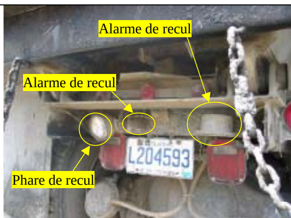
Figure 6 : Arrière d'un camion à benne
