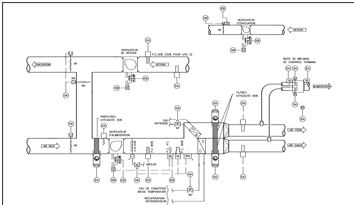
Figure 3.20 SCHÉMA INDICANT LES POINTS DE CONTRÔLE D'UN SYSTÈME CVCA À DOUBLE CONDUIT.
