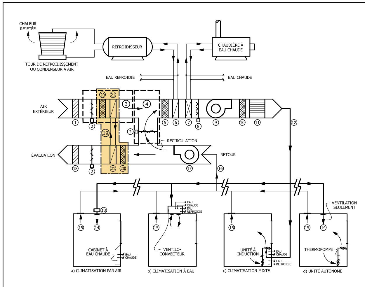
Figure 1 SCHÉMA DES TYPES DE SYSTÈMES CVCA
