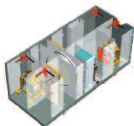
1.24 Récupération à roue thermique
