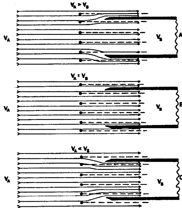
FIGURE 7: TRAJECTOIRE DE L'AIR (—) ET DES PARTICULES (-.-.) À L'ENTRÉE (10)
