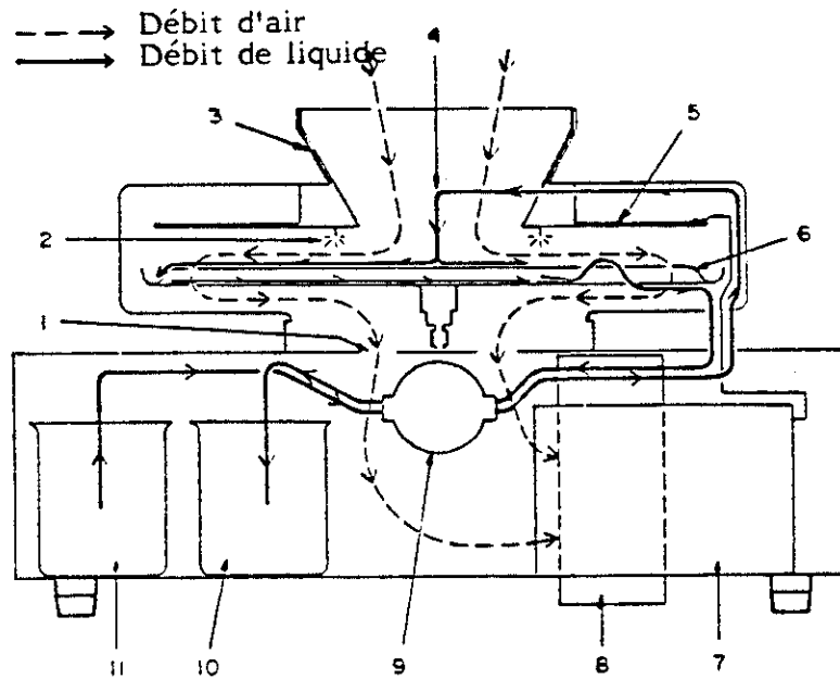
FIGURE 17: ÉCHANTILLONNEUR À LARGE VOLUME (9)
