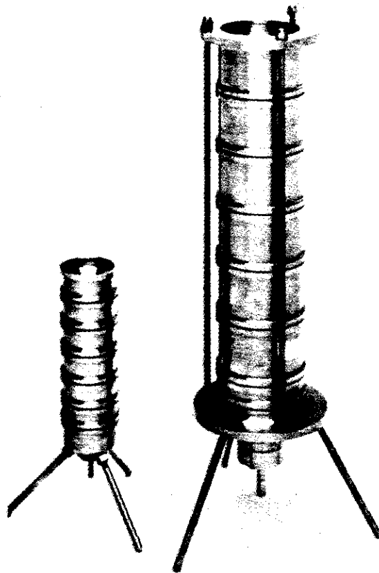
FIGURE 11: IMPACTEUR CASCADES MODIFIÉ (13)
