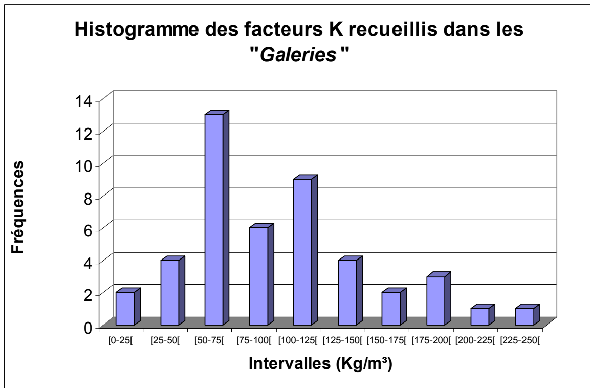
Graphique 1 : histogramme des facteurs K mesurés dans les grandes galeries
