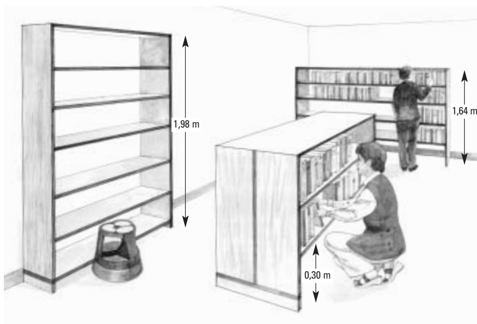
Hauteurs recommandées pour les rayonnages
