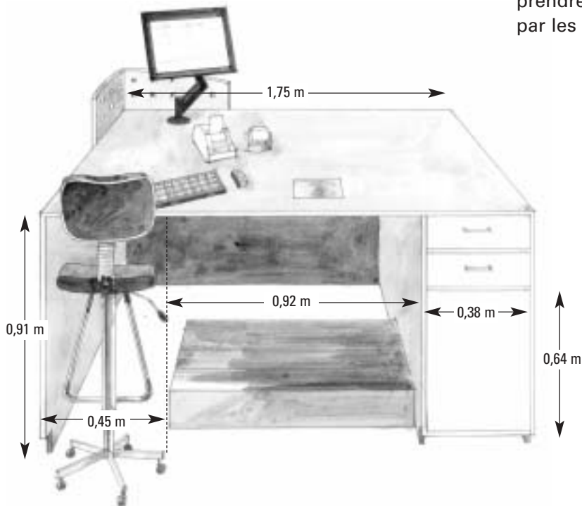
Dimensions du module de travail en position haute.
