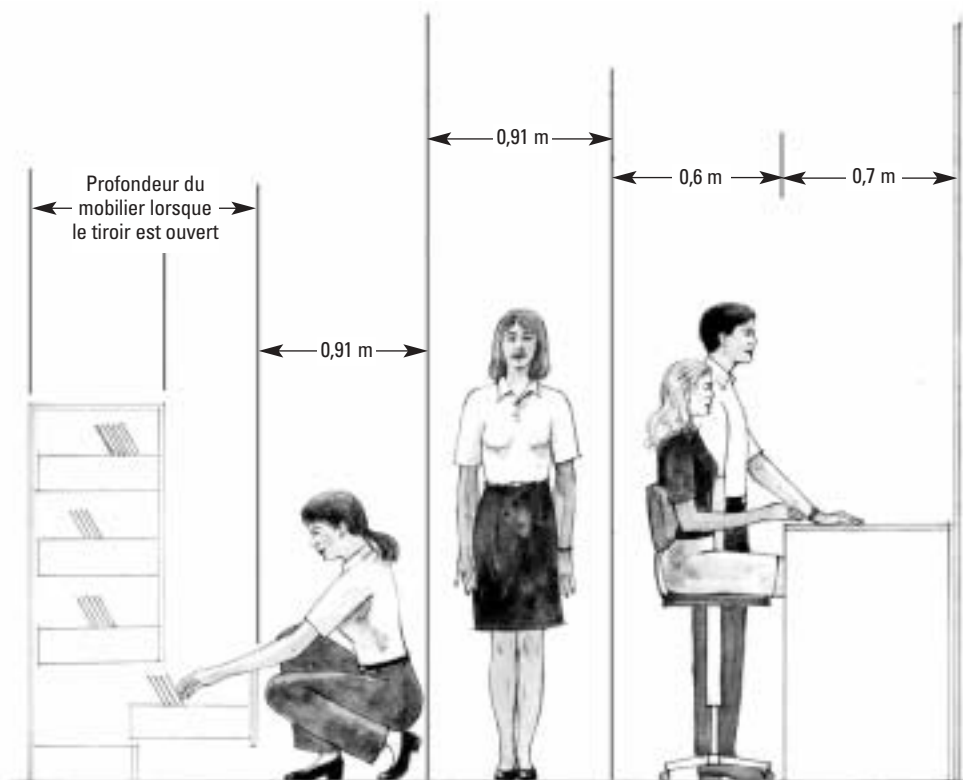
Dégagements nécessaires pour diverses zones d'activité.
