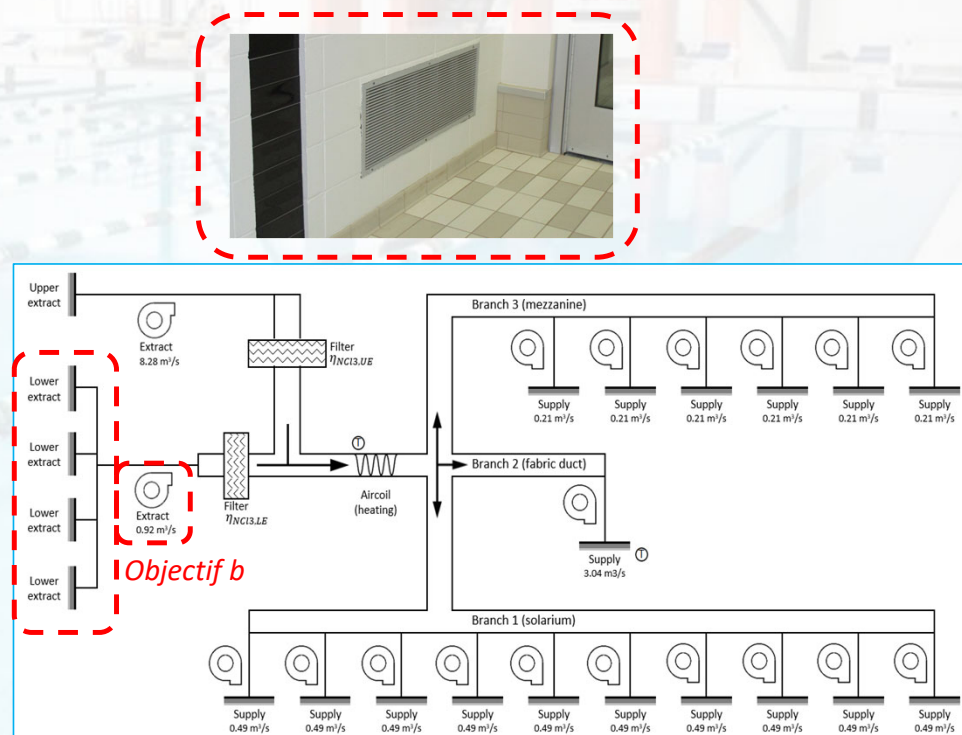
Système modifié avec l'ajout de 4 grilles d'extraction basse
