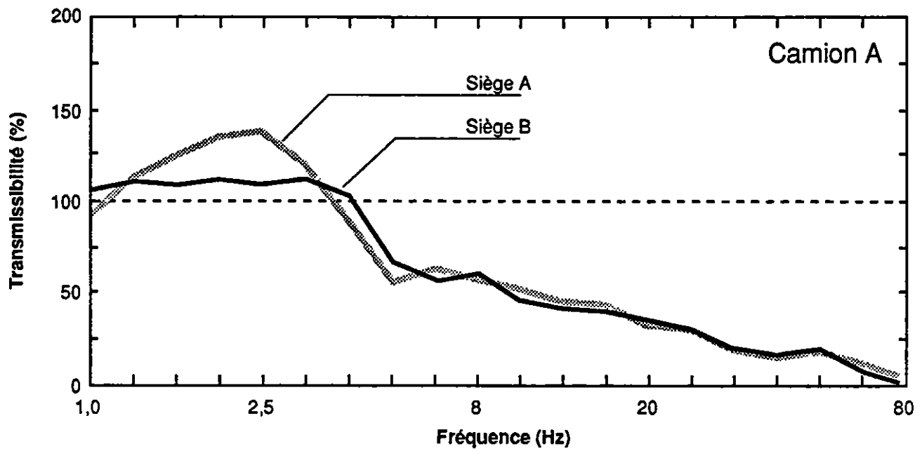
Figure 9: Courbes de transmissibilité des vibrations verticales mesurées sur le camion A
