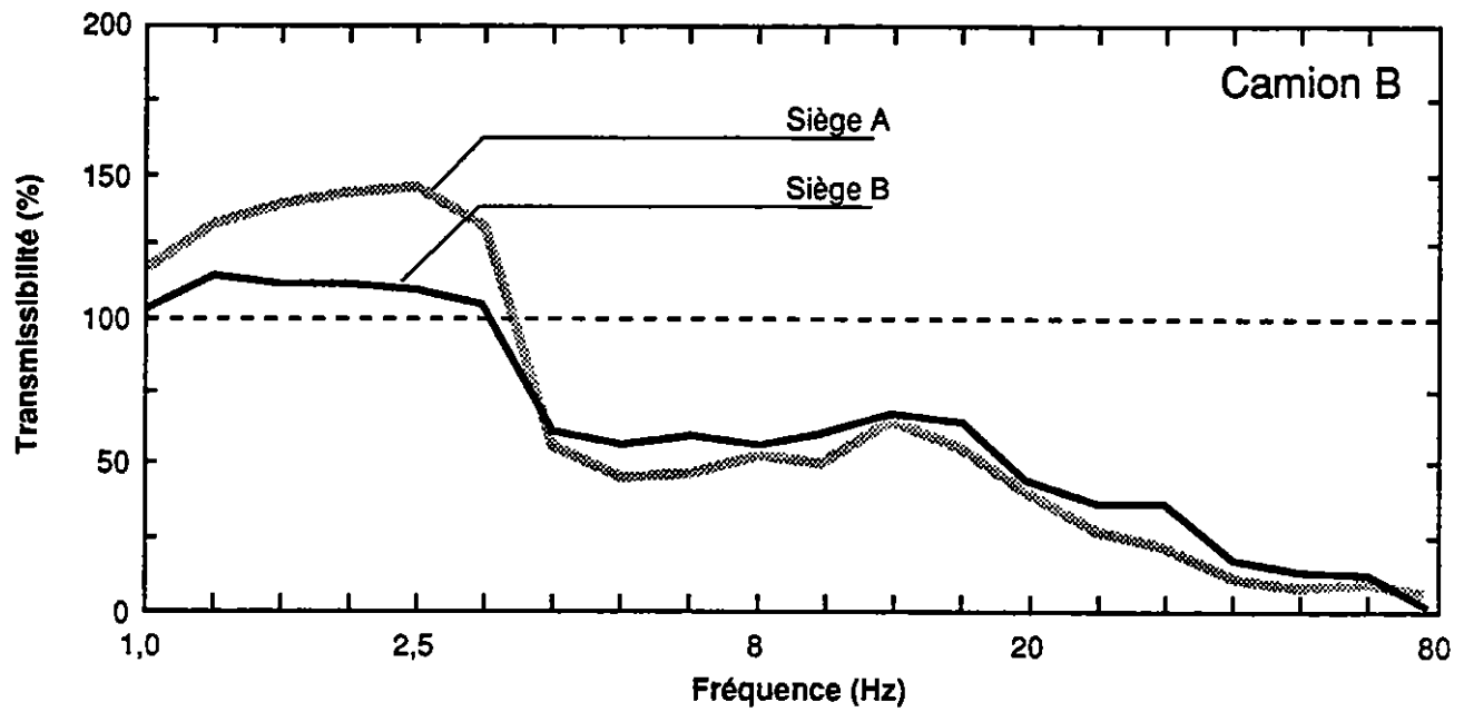
Figure 10: Courbes de transmissibilité des vibrations verticales mesurées sur le camion B
