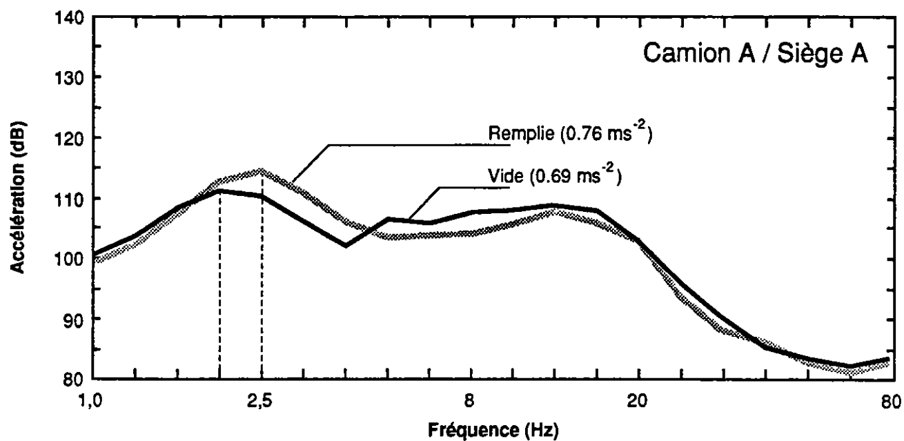
Figure 5: Spectres en fréquence des vibrations mesurées en direction verticale pour la combinaison camion A / siège A lorsque la citerne est vide et remplie
