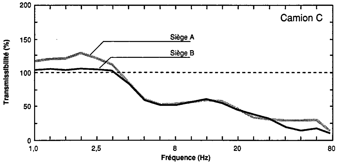
Figure 11: Courbes de transmissibilité des vibrations verticales mesurées sur le camion C
