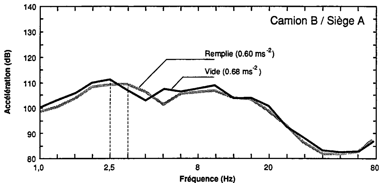
Figure 7 : Spectres en fréquence des vibrations mesurées en direction verticale pour la combinaison camion B / siège A lorsque la citerne est vide et remplie
