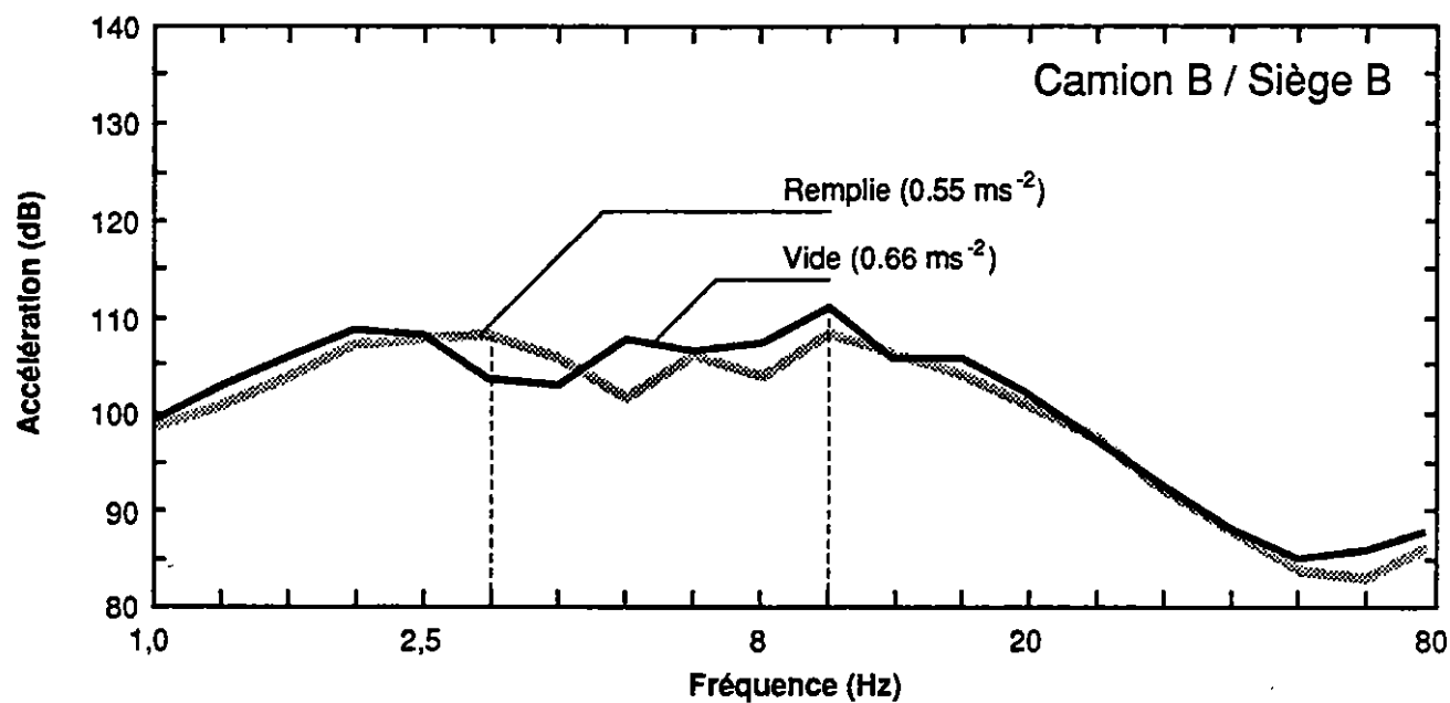
Figure 8: Spectres en fréquences des vibrations mesurées en direction verticale pour la combinaison camion B / siège B lorsque la citerne est vide et remplie
