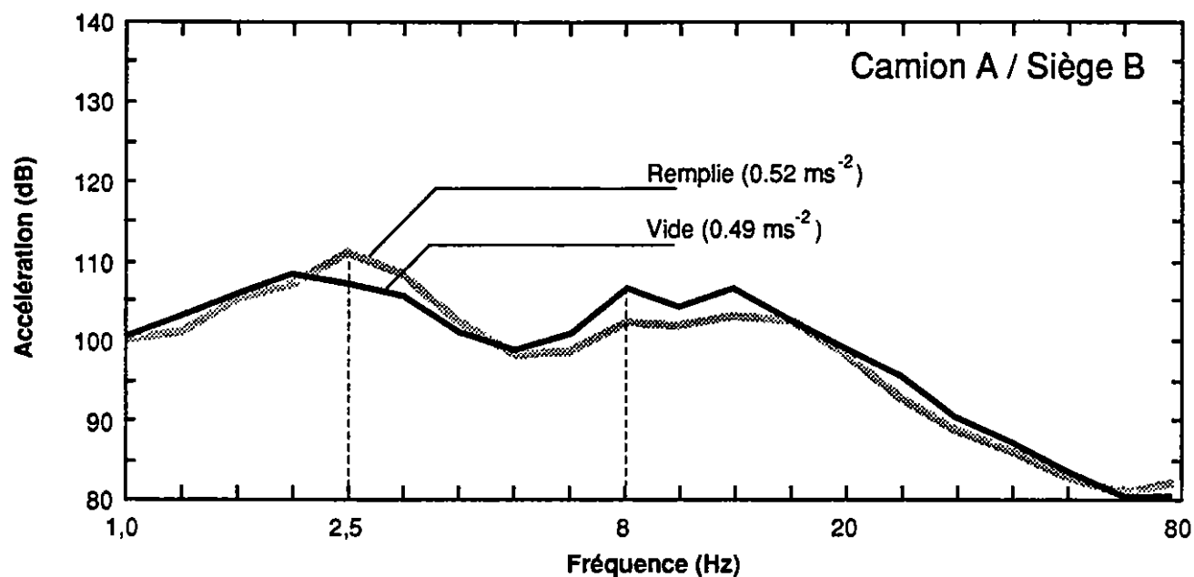
Figure 6: Spectres en fréquence des vibrations mesurées en direction verticale pour la combinaison camion A / siège B lorsque la citerne est vide et remplie
